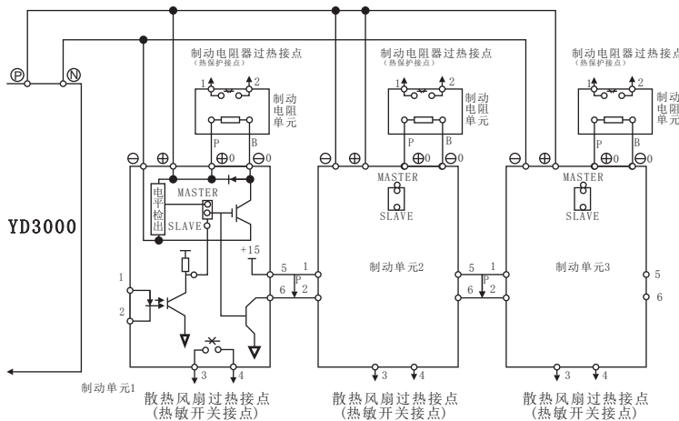
制动单元的并联连接
