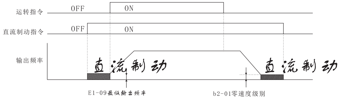
直流制动指令的时序图
