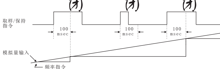
模拟量频率指令的取样/保持
