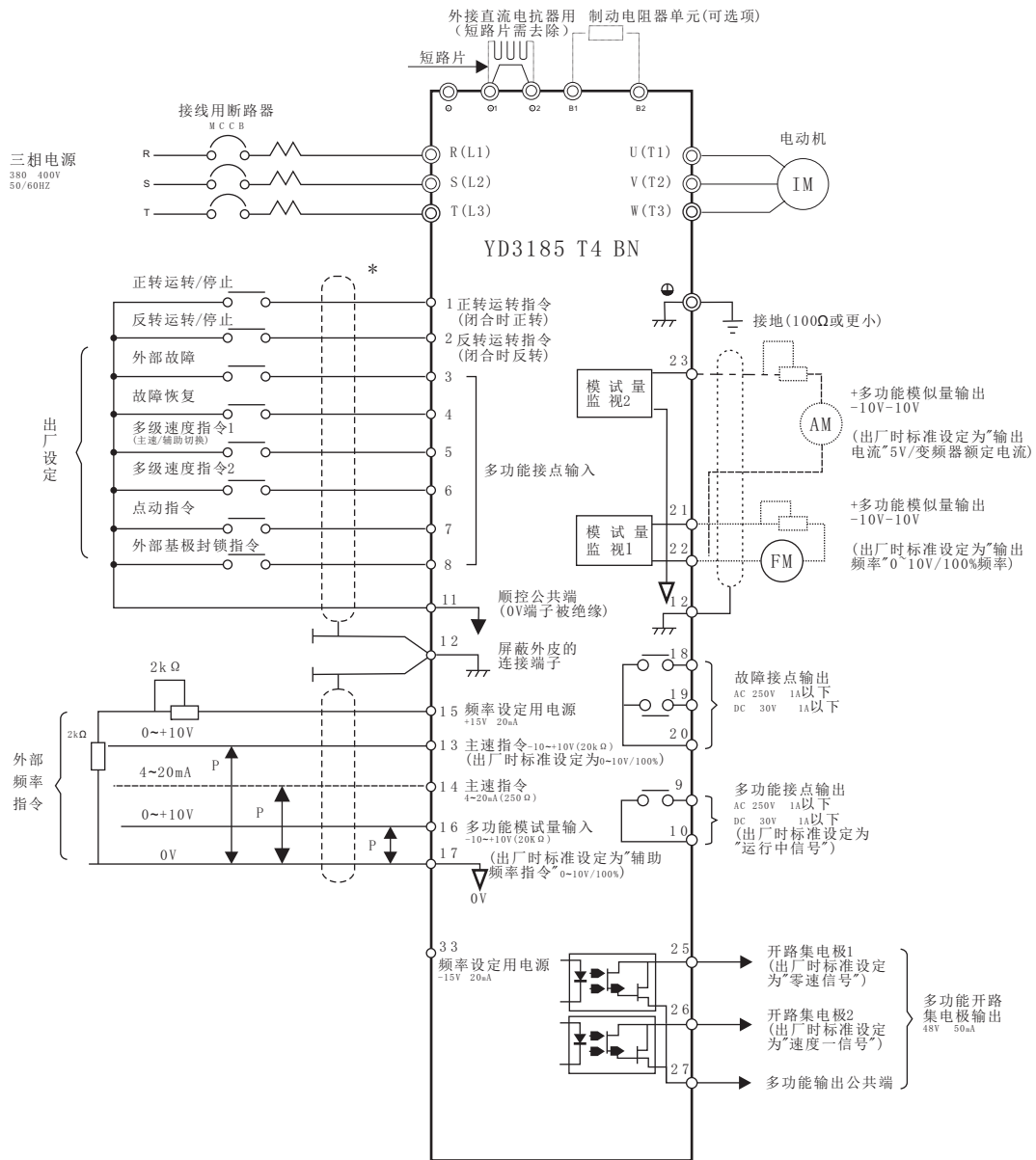
连接图(以YD3185 T4 BN 为例)
