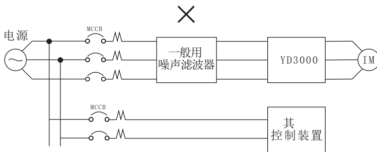
电源侧噪声滤波器的不正确设置举例
