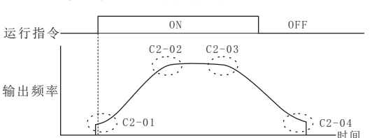
S字特性功能的设定
