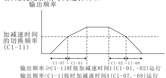
加减速时间的切换频率
